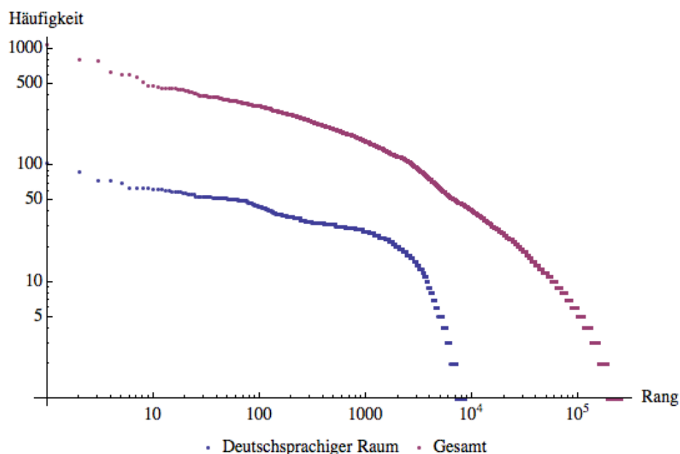
Abb. 4: Ressourcenwiederverwendung in LON-CAPA, Ressourcen ranggeordnet nach Wiederverwertungshäufigkeit (blau: deutschsprachiger Raum, rot: weltweit)
