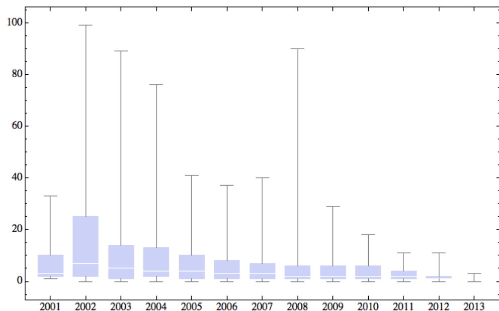
Abb. 6: Abhängigkeit des Hirsch-Indexes vom Zeitpunkt der ersten Veröffentlichung im System. Für jedes Jahr ist die Verteilung der H-Indices der Autorinnen und Autoren, die in diesem Jahr ihre erste Ressource veröffentlicht haben, als Box-Plot dargestellt.
